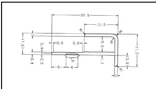
出隅ジョイナー5.5 LSD-27S7.3
