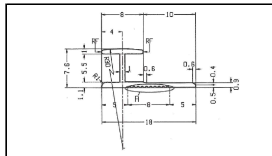
H型ジョイナー5.5 LSH-27S7.3
