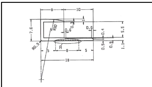
コ型ジョイナー5.5 LSM-27S7.3
