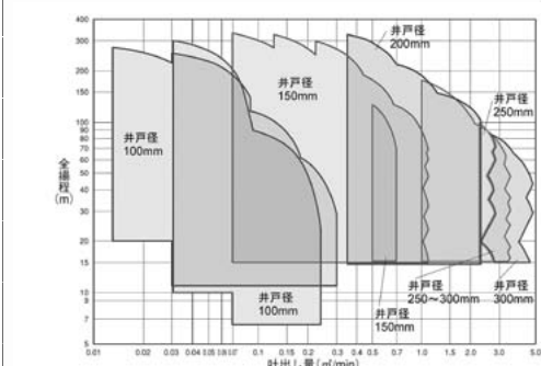
水中ポンプ④ <深井戸用水中ポンプ>
