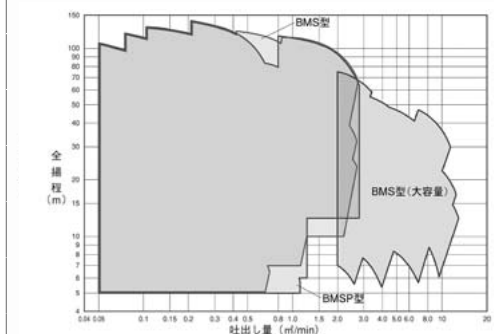
水中ポンプ⑤ <清水用水中ポンプ>
