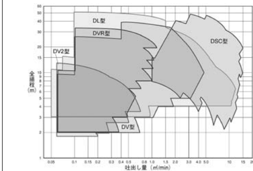
水中ポンプ③ <汚物・固形物用水中ポンプ>
