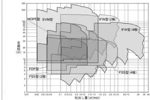
陸上ポンプ⑤ ■用途 ●冷温水循環 ●給湯 ●各種機械セット用 <ステンレス製ポンプ>
