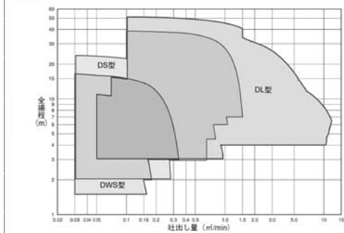
水中ポンプ① <汚水用水中ポンプ>
