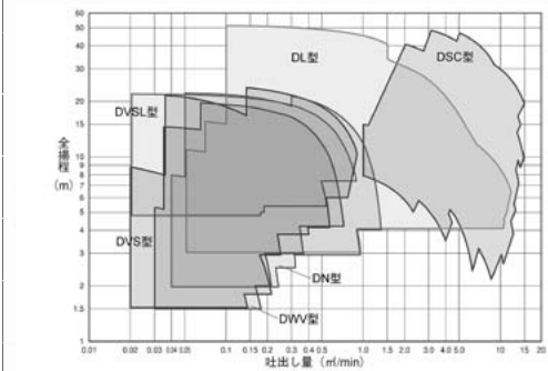
水中ポンプ② <汚物・雑排水用水中ポンプ>
