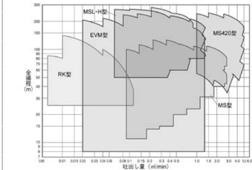
陸上ポンプ③ ■用途 ●一般給水・揚水 ●ボイラー給水 ●散水 <多段渦巻・渦流ポンプ>
