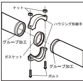
ハウジング形継手構成図
