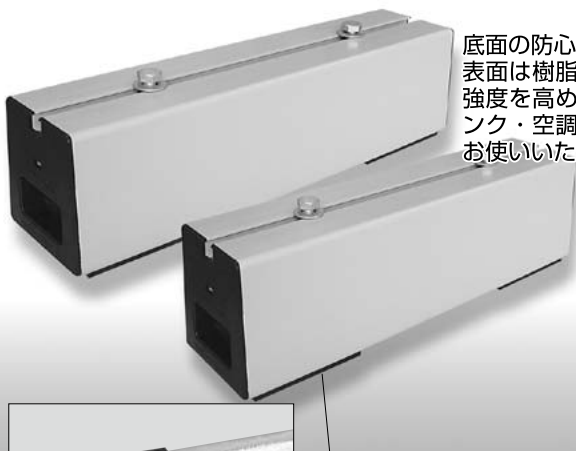
防振ゴム (ゴム厚5mm)
