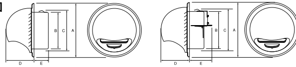
■寸法図
