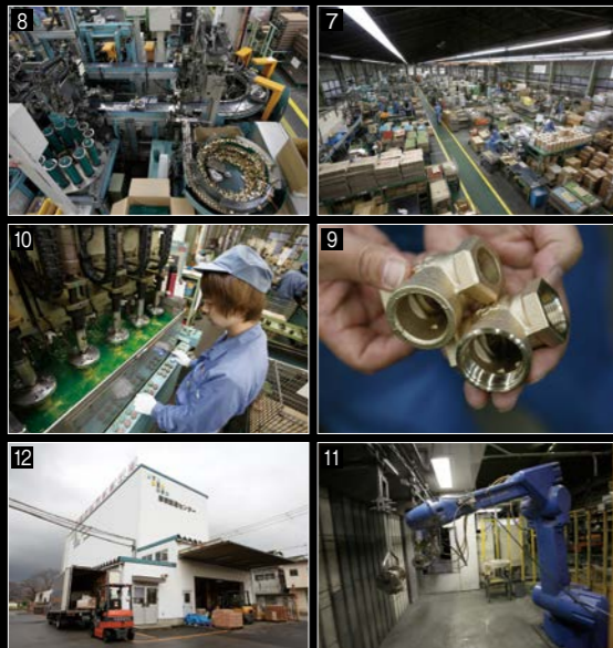
7 オートメーション化が進む加工工場。基本的にセット以外は全自動となっている。8 複雑な作業は人の手で加工が行われている。熟練職人の技術が光る。9 ネジ加工や穴開け加工など、自動機はさまざまな加工に対応している。10 検査工程は、自動検知検査機の判定と並行し、気泡が出ないかと人による目視判定により検査を行い、「後工程はお客様」をモットーに全品検査が行われ、梱包され配送センターへと送られる。11 鑄鉄バルブやダクタイルバルブはロボットによる塗装が行われる。12 出荷用の倉庫も彦根工場内に完備。
