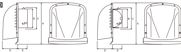
■寸法図
