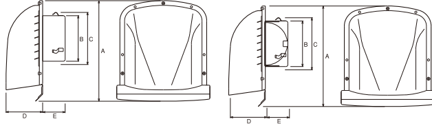
■寸法図
