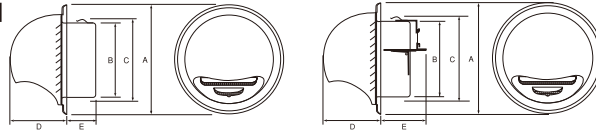
■寸法図
